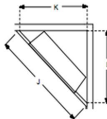
Rohbau Eckmaße
