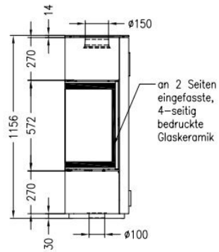
Vorderansicht M~1:20
