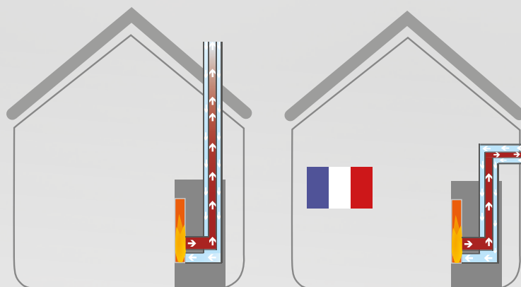
Installatievoorbeeld met coaxiale rookgasafvoer en externe luchtinlaat.
