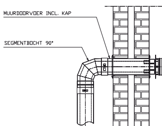
4. Muurdoorvoer met kap
