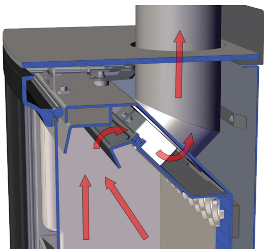
Purevision Actieve Klep Systeem Dicht
