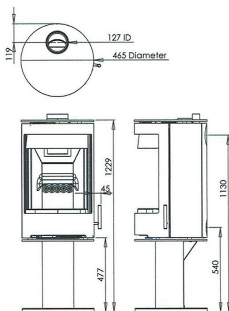
Purevision Rond houtkachel op hoog voetstuk
