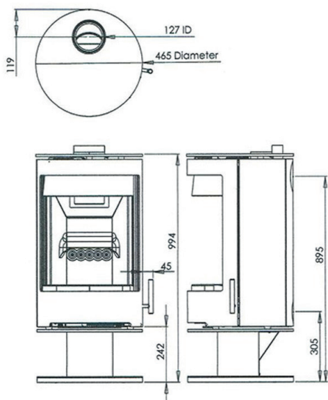
Purevision Rond houtkachel op laag voetstuk
