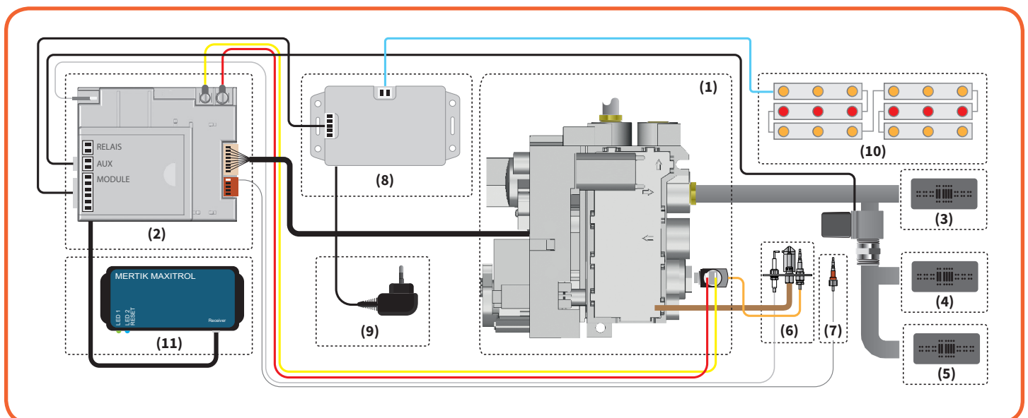
Afbeelding 9.1 - Electronisch schema van de Summum 70
