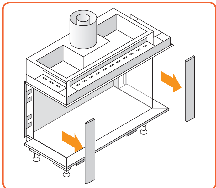
Afbeelding 10.2 - Verwijderen van de zij sierlijsten
