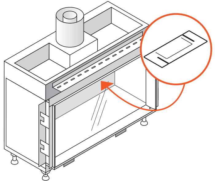
Afbeelding E.1 - Positie Rookgasbegrenzer Summum 70
