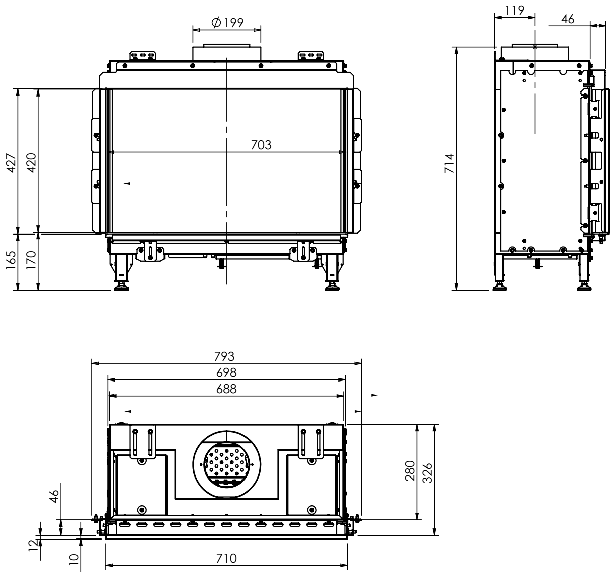
Afbeelding I.1 - Lijntekening Summum 70 F
