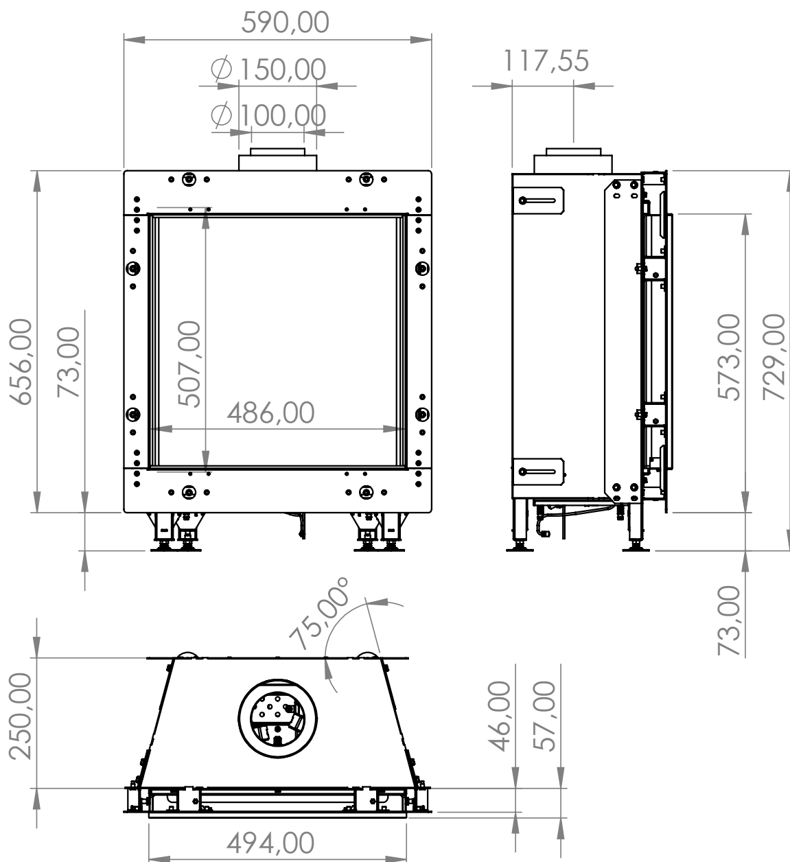
Afbeelding I.1 - Lijntekening Cupido 50
