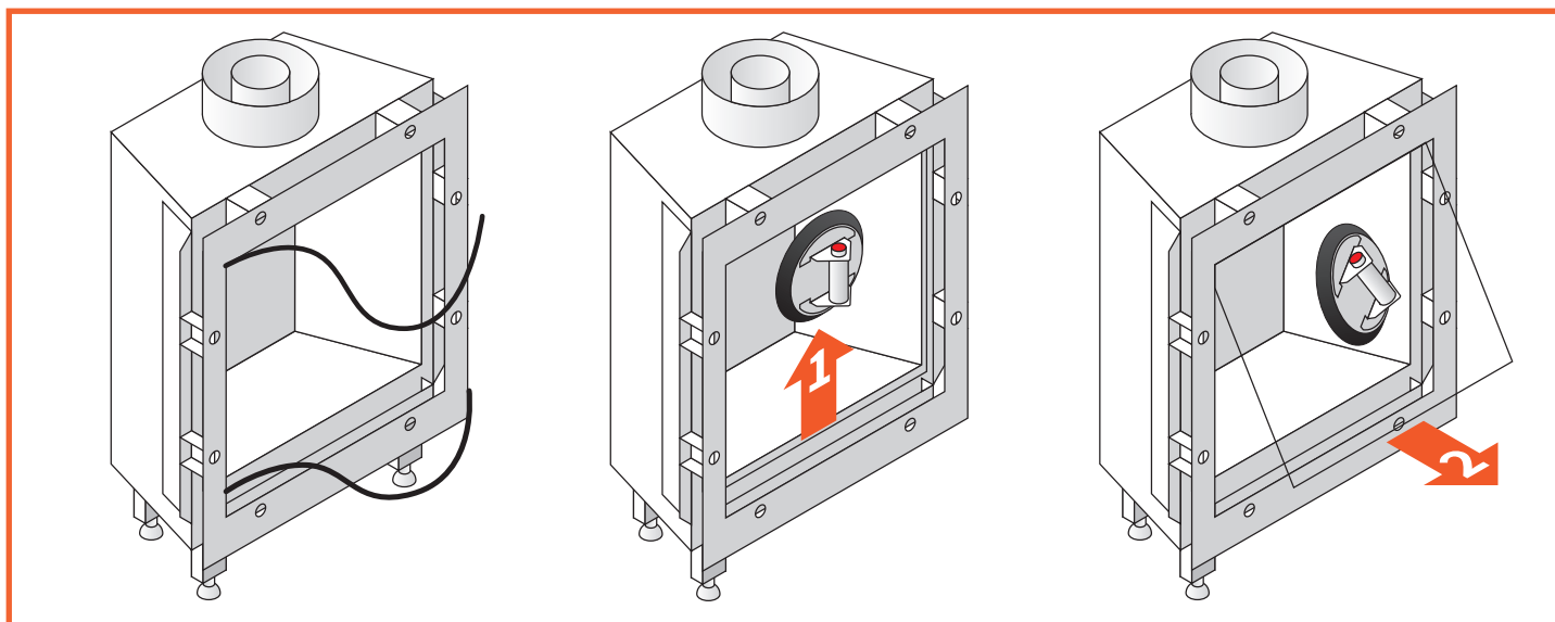
Afbeelding 10.6 t/m 10.8 - Uithalen van de glaskoorden en het glas
