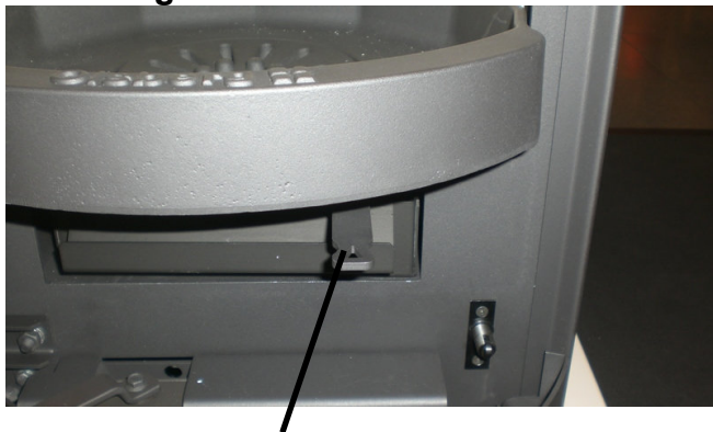
Regelhendel voor het vuurrooster
